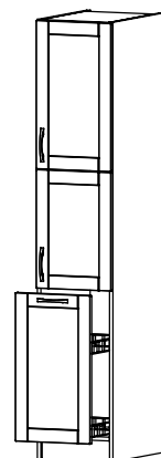
SK-40/200-c SK-40/212-c
